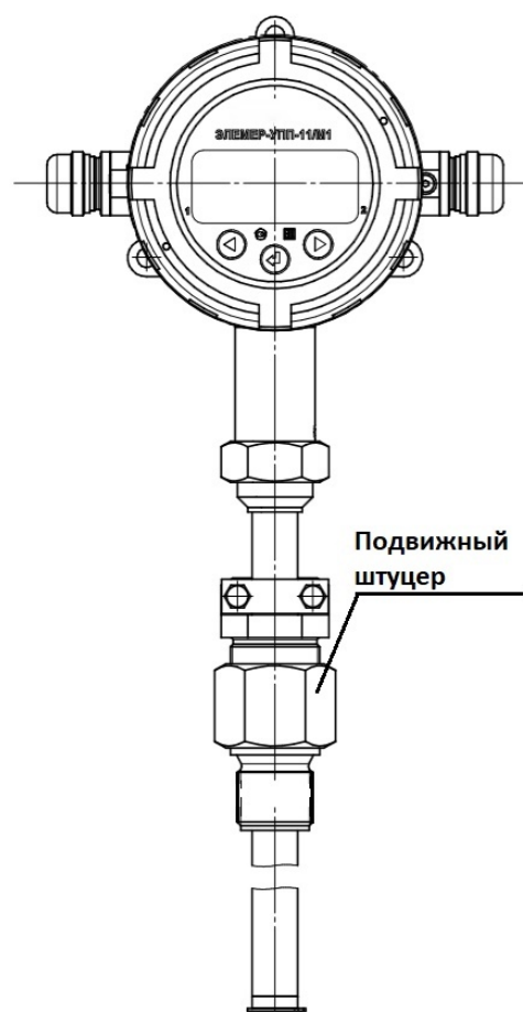
Рис.2 ЭЛЕМЕР-УПП-11/M1L с подвижным штуцером, индекс заказа «ПШ».
